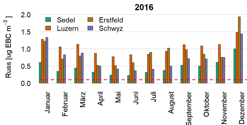
Abbildung 26: Monatsmittelwerte für das Jahr 2016. Zum Dezember 2016 schreibt MeteoSchweiz: «Die Dezembertemperatur in den Tieflagen der Alpennordseite und der Alpentäler (blieb) verbreitet 0.4 Grad bis 1.7 Grad unter der Norm 1981–2010». 54 Dies kann die erhöhten Werte durch intensive Heiztätigkeiten erklären.
