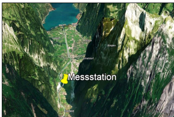
Abbildung 49: Die Messstation «Erstfeld, A2 Uri» in der topografischen Ansicht. Die Höhen sind um das Dreifache verstärkt. 56
