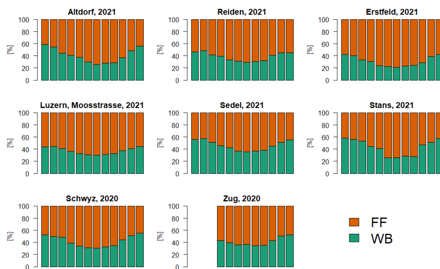
Abbildung 67: Ergebnisse aus dem Aethalometer-Modell: Relative Russwerte, aufgeteilt in die Quellen «ff» (fossil fuel), welche auf Verkehr hindeuten, und «wb» (wood burning), welche auf Holzheizungen hinweisen.
